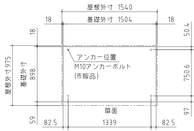
ベタ基礎図
