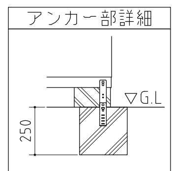
仕様図
